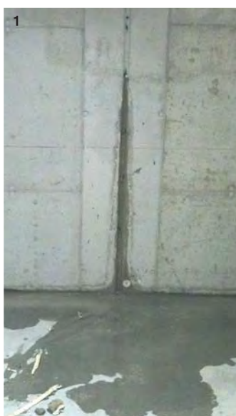
Foto 1) Lesione con fuoriuscita di acqua in spinta idraulica - Foto 2) Predisposizione dei fori per i packer di iniezione - Foto 3) Fissaggio dei packer a tenuta nei fori Foto 4) Iniezione con pompa elettrica della resina idroespansiva elastica.
