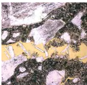
Foto 1) Campionature di valutazione con carotaggi dalla matrice in calcestruzzo delle strutture interrate sotto falda marina del Terminal 3 dell'aeroporto di Singapore Foto 2) Presenza di cristalli di differente forma e dimensione lungo una fessurazione: essi sigillano completamente la crepa (cristalli C-S-H, Silicato di Calcio Idrato) Foto 3) Ingrandimento "BEI" (backscattered electron image), mostra la crescita cristallina all'interno di una microfessurazione Foto 4) Particolare ulteriormente ingrandito della "BEI" mostra le tipologie di cristalli: sottili e oblungi, fini ed aghiformi.
